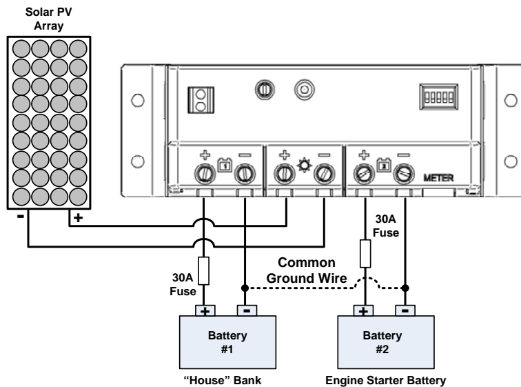
Abbildung 5: Typischer Bootsverkabelungs-Schaltplan
