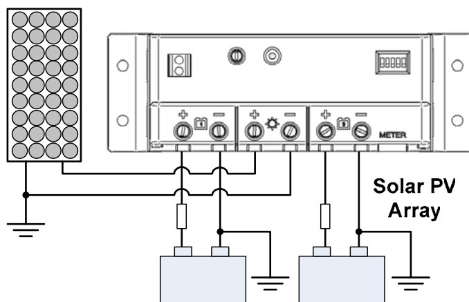
Abbildung 6: Verkabelungsschaltplan für unbewegliche Installationen
